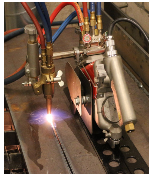
Прямой рез с рельсом IK-93
