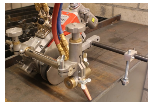
Для резки с краю листа с направляющим роликом
