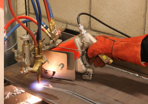
Направление ручной резки
